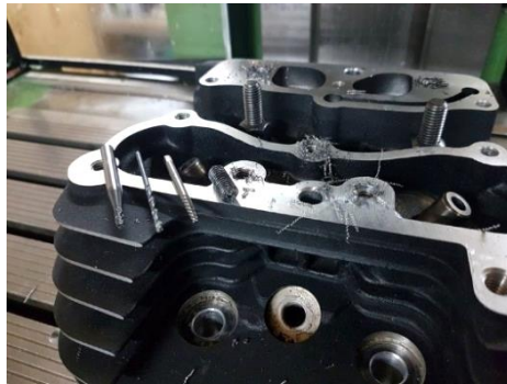
Reparatur eines Harley Davidson Zylinderkopf
